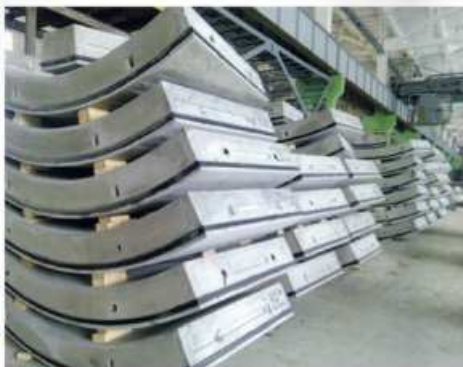
Готовые бетонные элементы для строительства тоннелей
